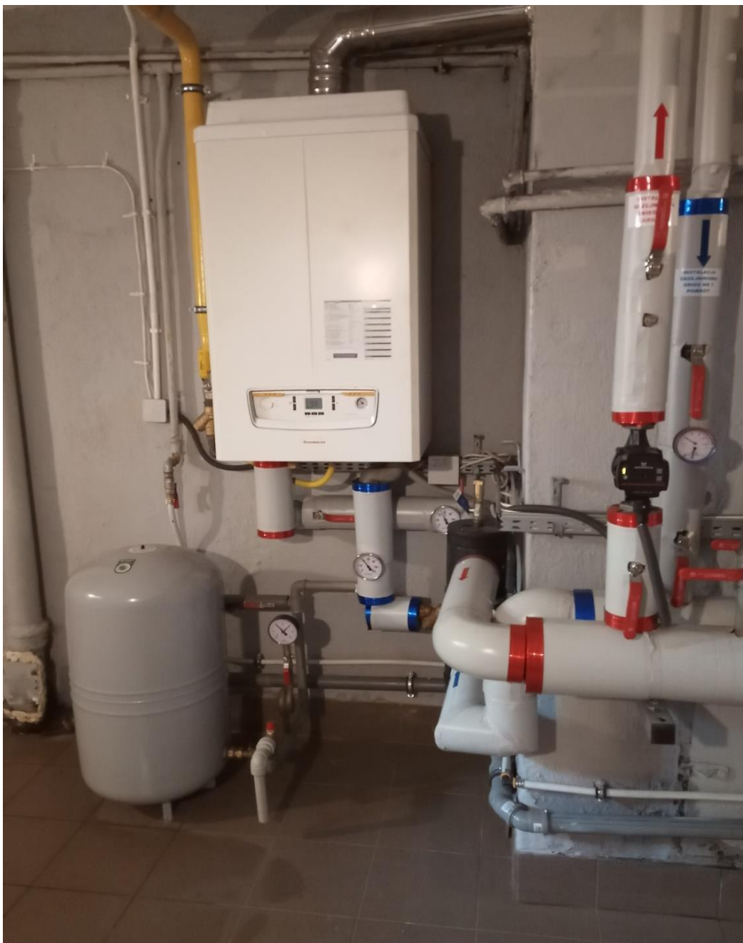
Nowa kotłownia zasilana gazem ziemnym
